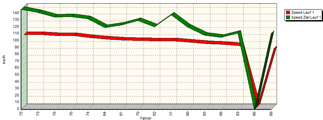
Speed-Diagramm Lauf 1
